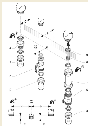
Opalia F 14 E
